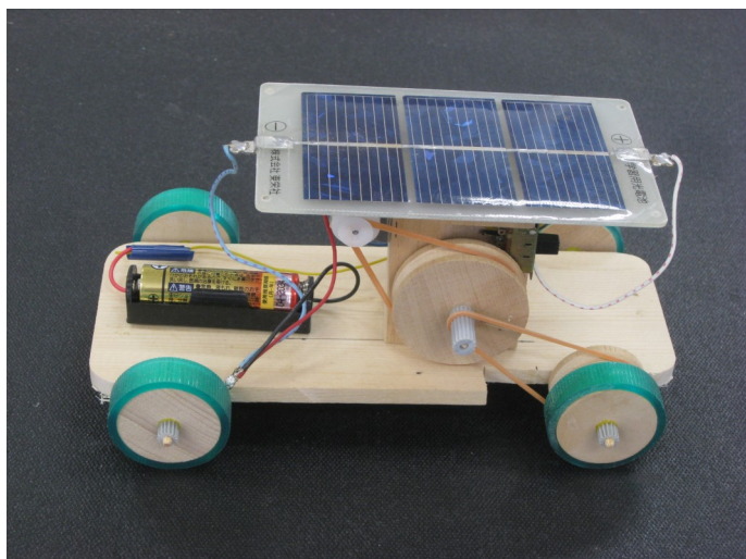
エコなハイブリッドソーラーカー
